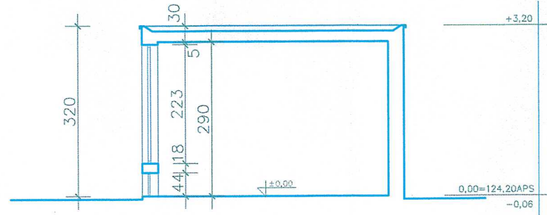
PRESJEK A-A
